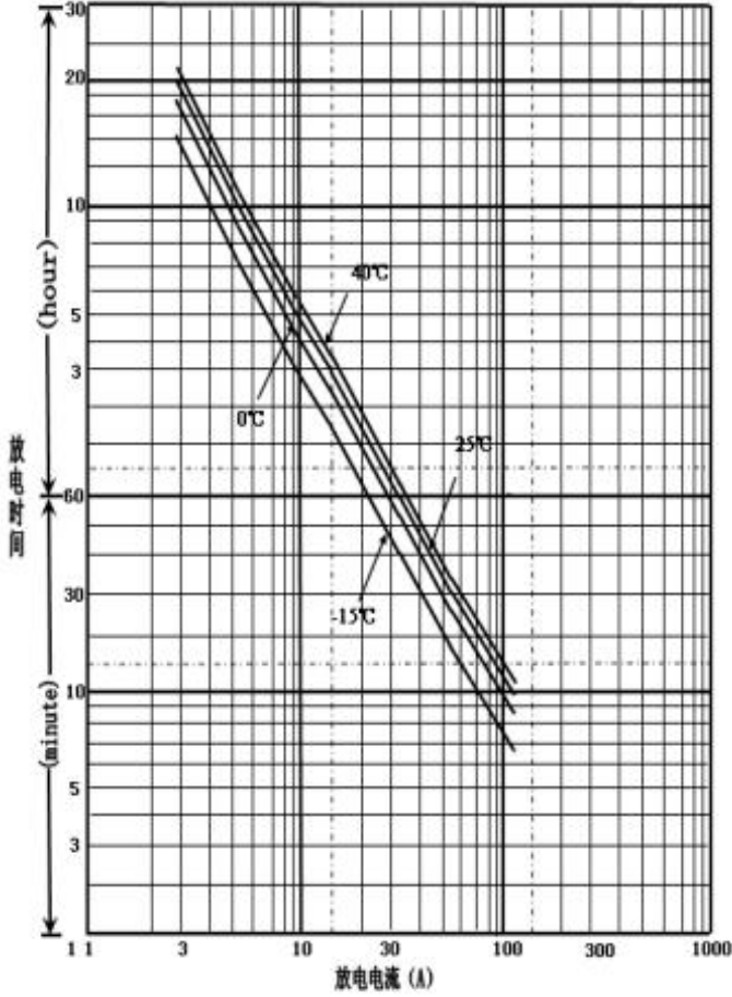
放电特性
